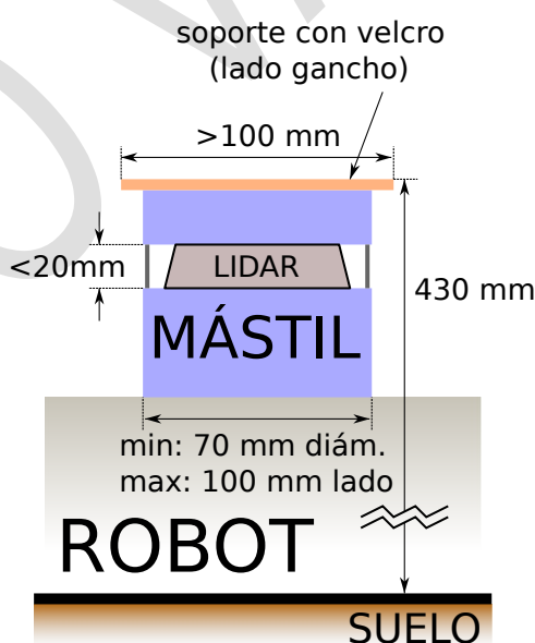
Figura 3: mástil con LIDAR incorporado
