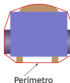
Figura 2: envolvente convexa
